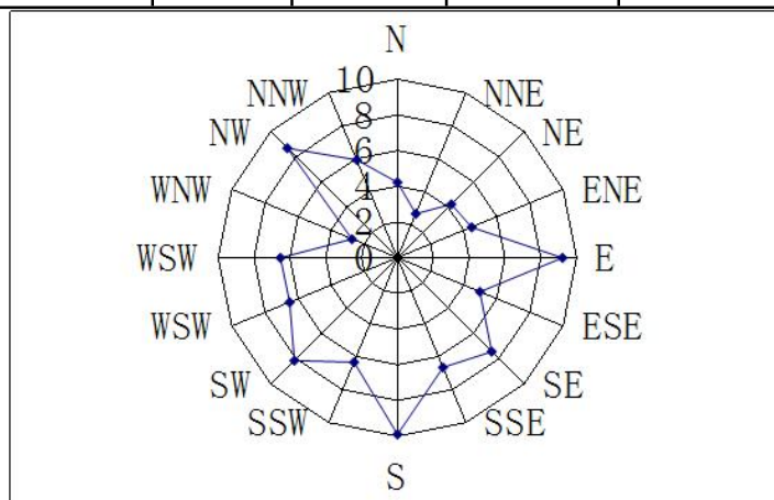
图 3.1-1 风玫瑰图
