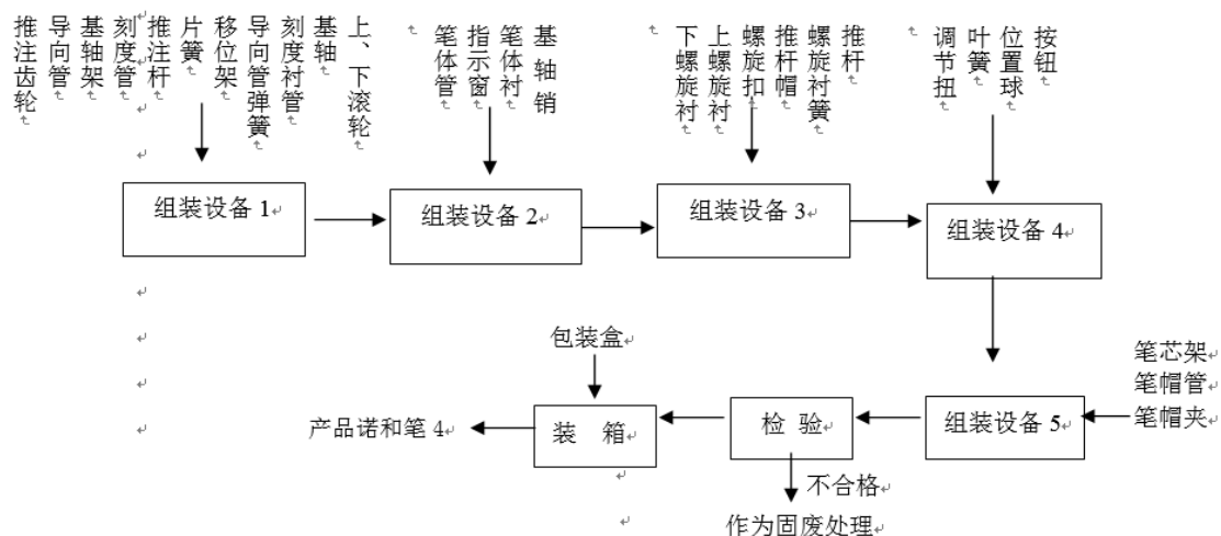
图 2.2-2 诺和笔 4 组装线生产工艺及污染流程图
